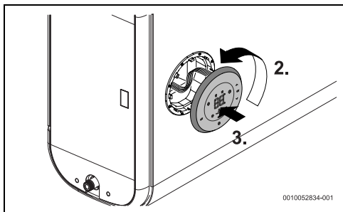
Фиг. 13 Завъртете и фиксирайте дисплея
