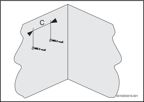
Фиг. 10 Фиксиращи винтове
