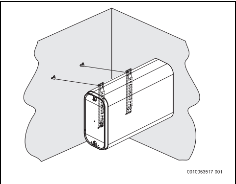
Фиг. 11 Хоризонтална инсталация (стенен монтаж)
