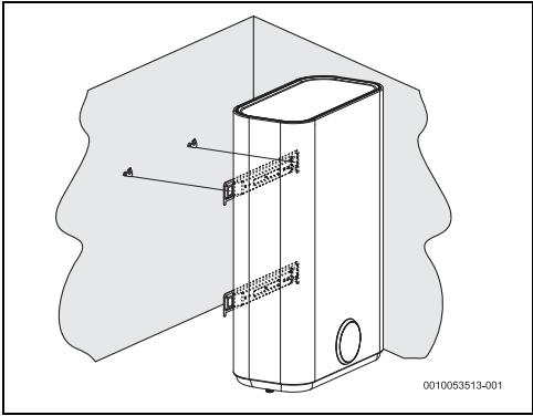
Фиг. 9 Вертикална инсталация (стенен монтаж)
