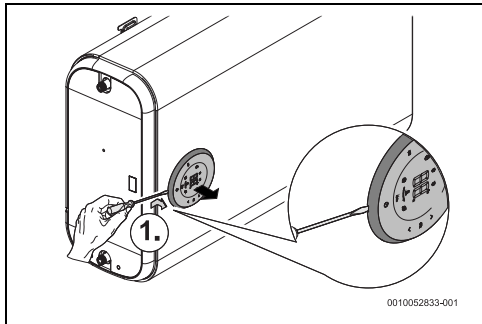
Фиг. 12 Демонтаж на дисплея
