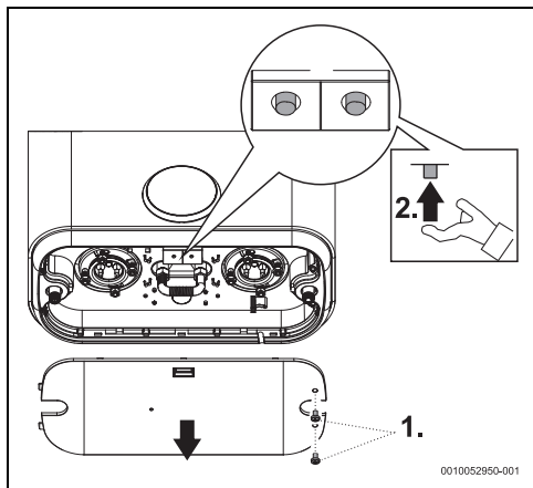
Фиг. 16 Предпазен термостат
